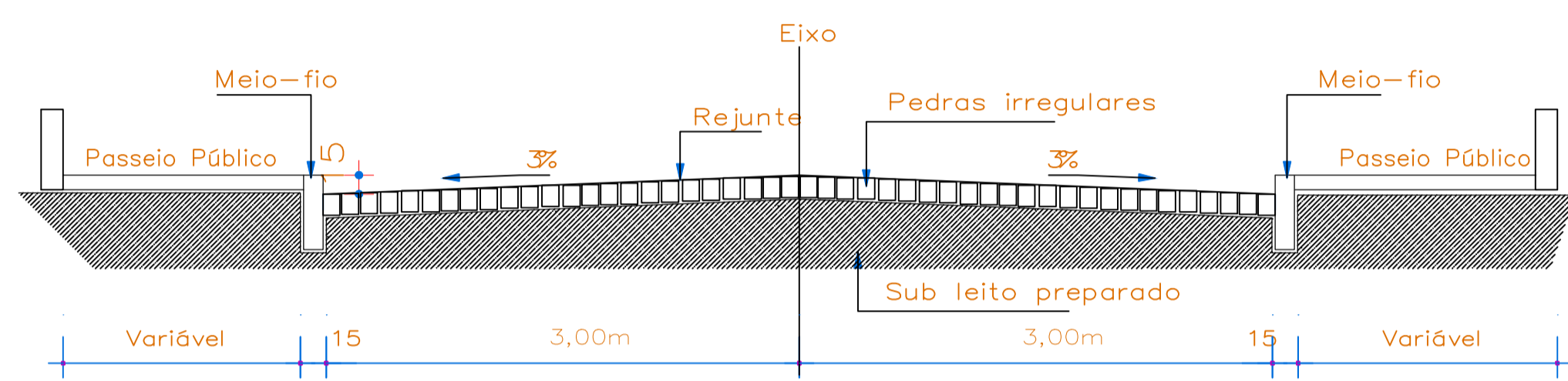
PERFIL TRANSVERSAL
