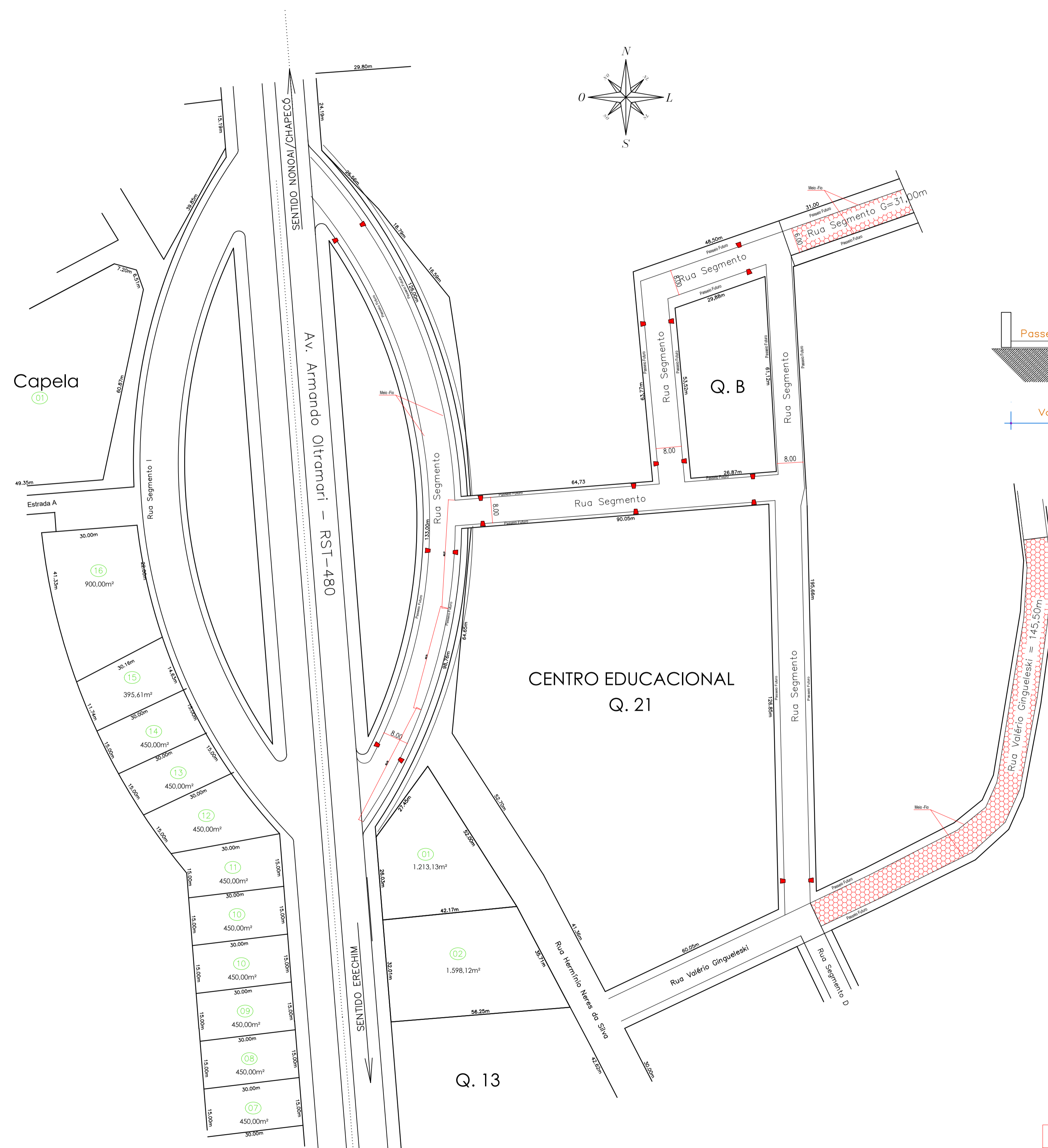
PLANTA DE PAVIMENTAÇÃO
